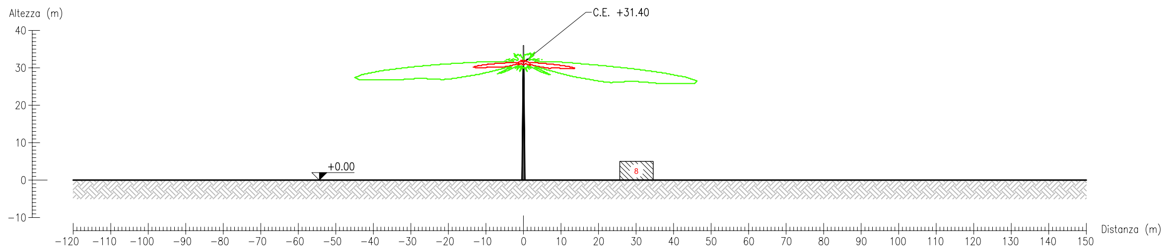
SEZIONE SETTORE 3 – 280° Campo 6 e 20 V/m – Vista Unica Scala 1:1000
