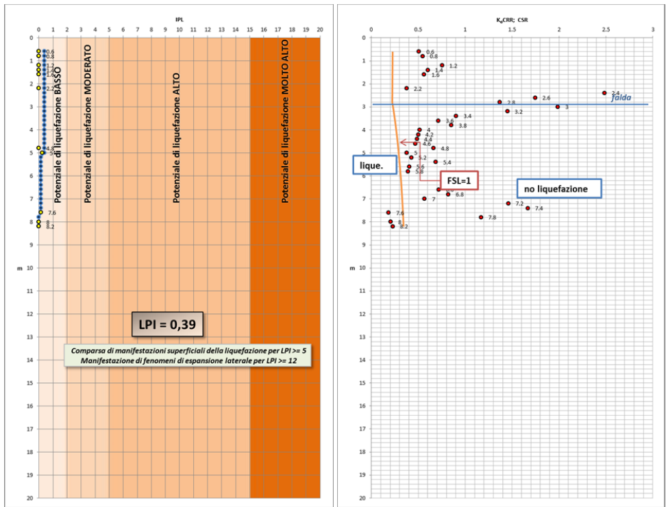
Risultati grafici del calcolo dell'Indice di Potenziale Liquefazione lungo la CPT2 dell'ambito 39 ASP.b nello scenario di Risposta Sismica Locale con interfaccia risonante a -13 m.
