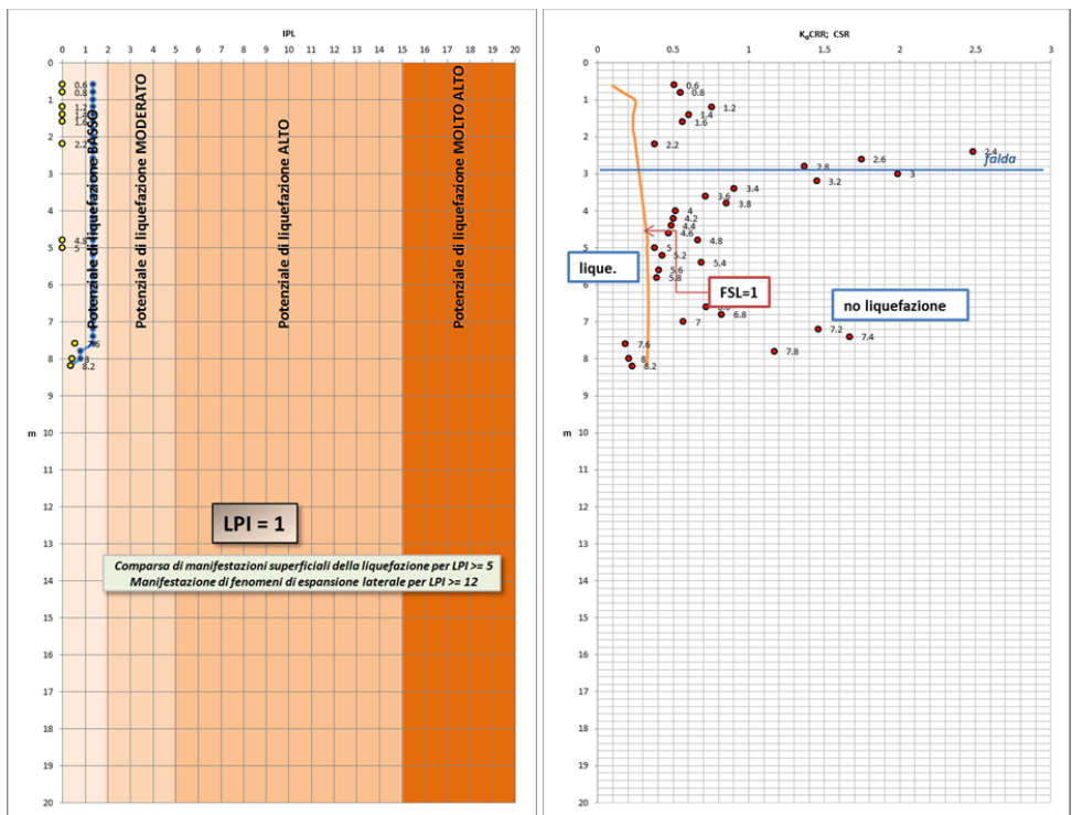
Risultati grafici del calcolo dell'Indice di Potenziale Liquefazione lungo la CPT2 dell'ambito 39 ASP.b nello scenario di Risposta Sismica Locale con bedrock sismico a -120 m.
