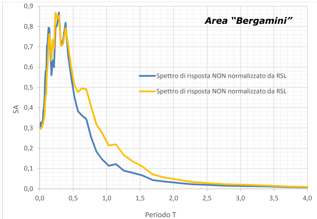
Figura 21 - Confronto tra gli spettri di risposta visco-elastici, NON normalizzati, ottenuti da analisi di risposta sismica locale eseguita presso l'area "Bergamini" considerando il bedrock sismico a -120 m (linea arancio) e l'interfaccia risonante a -15 m (linea blu).
