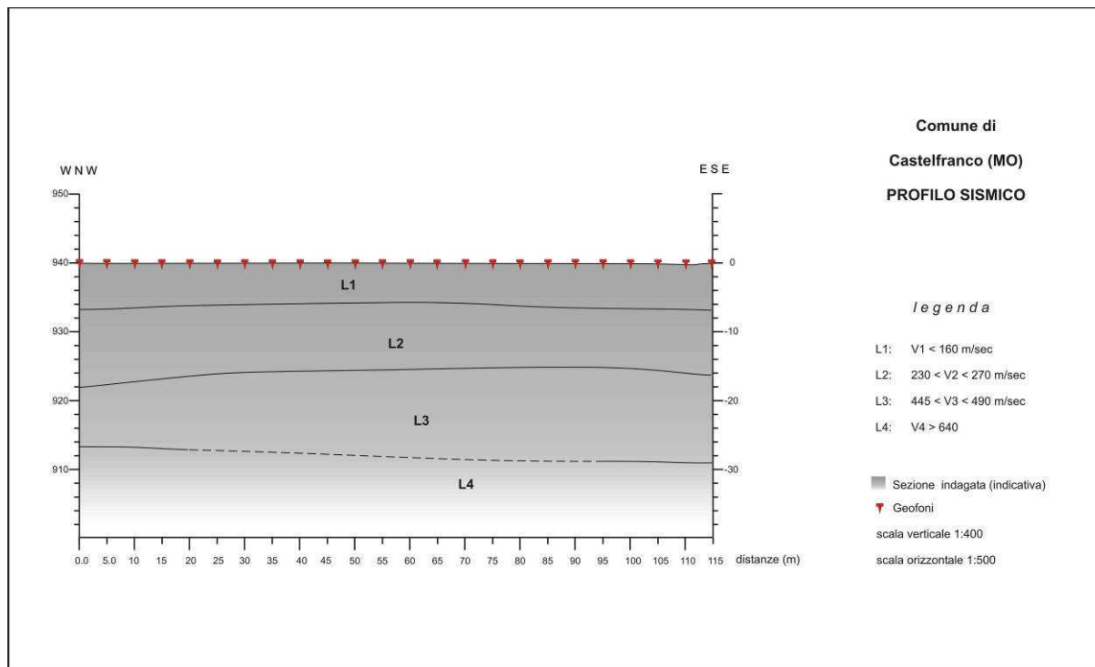
Figura 30 - Profilo sismostratigrafico.
