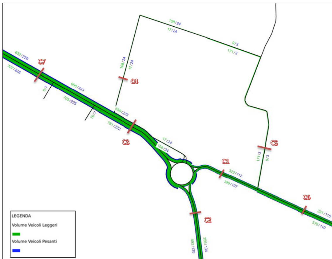
Img. 4.1 - Flussi di traffico nello scenario futuro – ora di punta della sera
