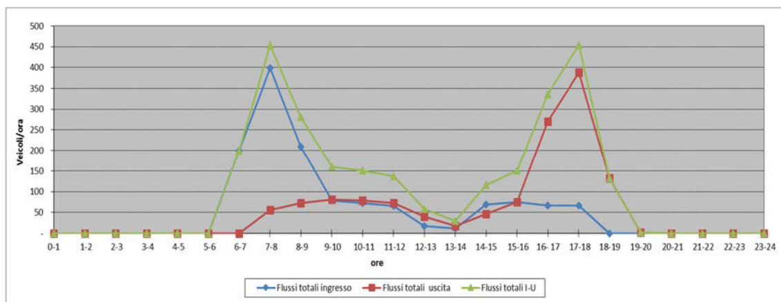
Graf. 3.1 - Distribuzione oraria dei flussi veicolari in ingresso-uscita dai due ambiti 50 ANP e 58 ANP
