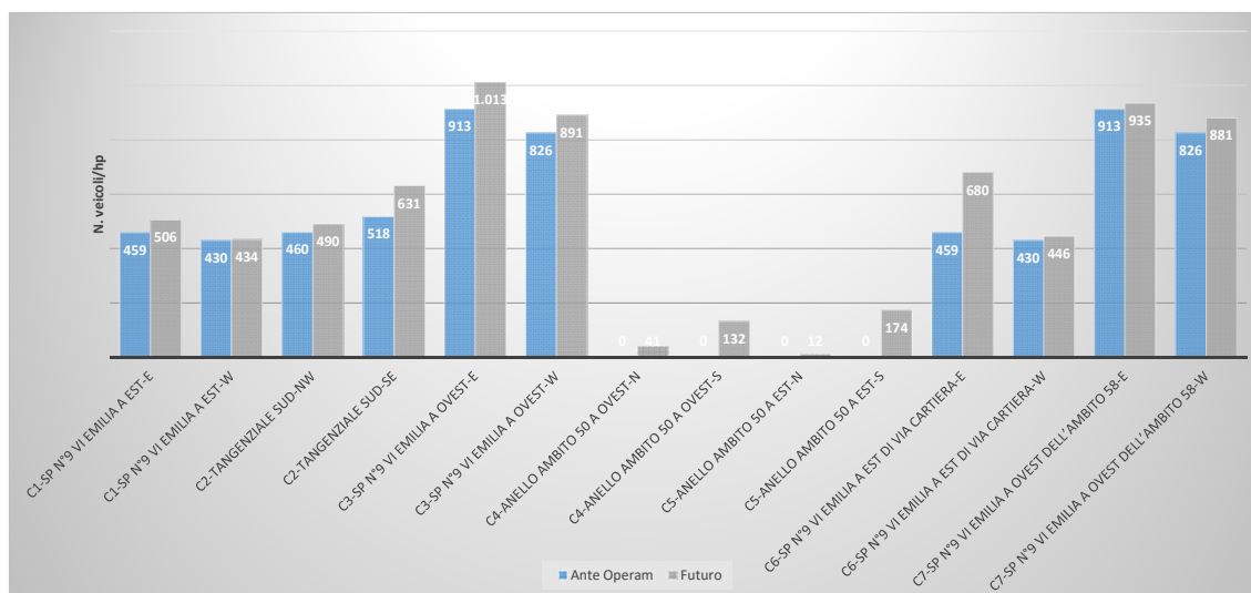
Graf. 4.1 - Flussi di traffico sulle sezioni di controllo nello scenario futuro e nello scenario ante operam (ora di punta della sera)
