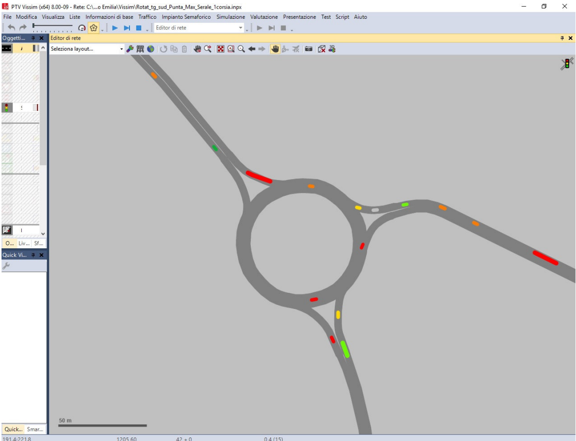
Img. 5.2 - Il modello di microsimulazione della rotatoria nello scenario ante operam
